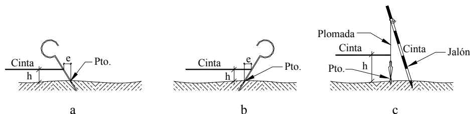
Figura 3.7. Error de verticalidad
